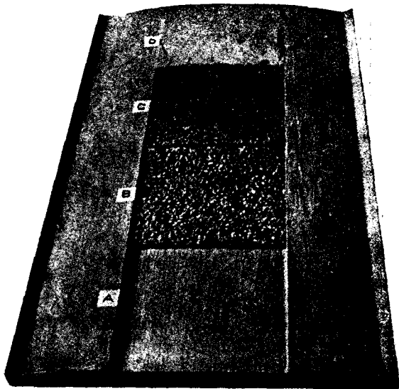
Фиг. 34. Модель устройства шоссеиной одежды; А — подготовка полотна; В — нижний слой из крупного (6 см) щебня; С — засыпка мелочью (меньше 2 см); D — гладкая поверхность укатанного шоссе.
