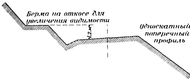
Фиг. 171. Срезка бермы на откосе выемки для обеспечения видимости на закруглении.
