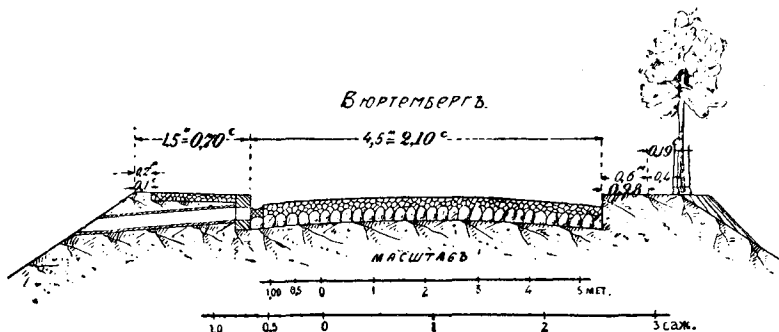
Фиг. 79. Шоссе с тротуарами на обочинах.
