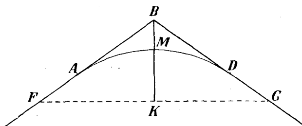
Фиг. 174. Определить величины срезка откоса для обеспечения видимости.
