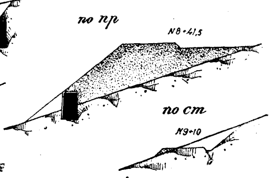
Фиг. 163. План, продольный профиль и поперечные профили серпантины.
