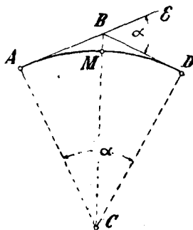
Фиг. 142. Разбивка кривой по касательным.
