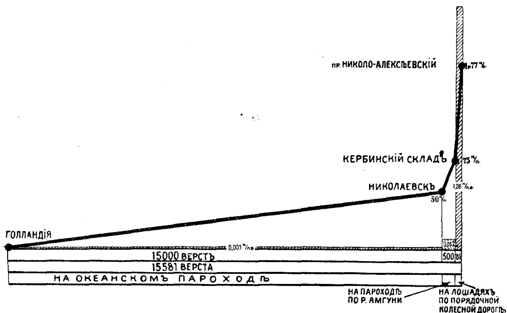
Фиг. 40. Стоимость перевозки 7\frac{1}{2} фут. драги (весом 16 000 пуд. ценою 100 000 руб.) летом 1910 г. из Голландии на Николо-Алексеевский прииск Амгунской К о (в коп./пуд. и коп./пуд. вер.).
