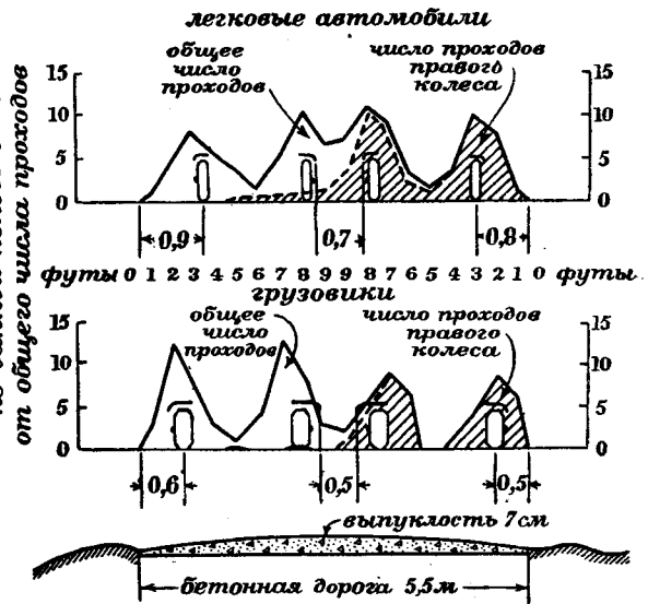
Фиг. 89 б. Движение на ширине 5,5 м.
