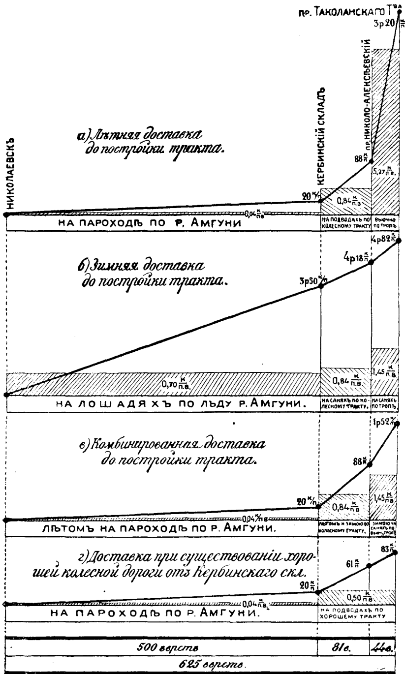
Фиг. 41. Фракты для грузов Амгунской К 0 в к/пд. и к/пд. вер.
