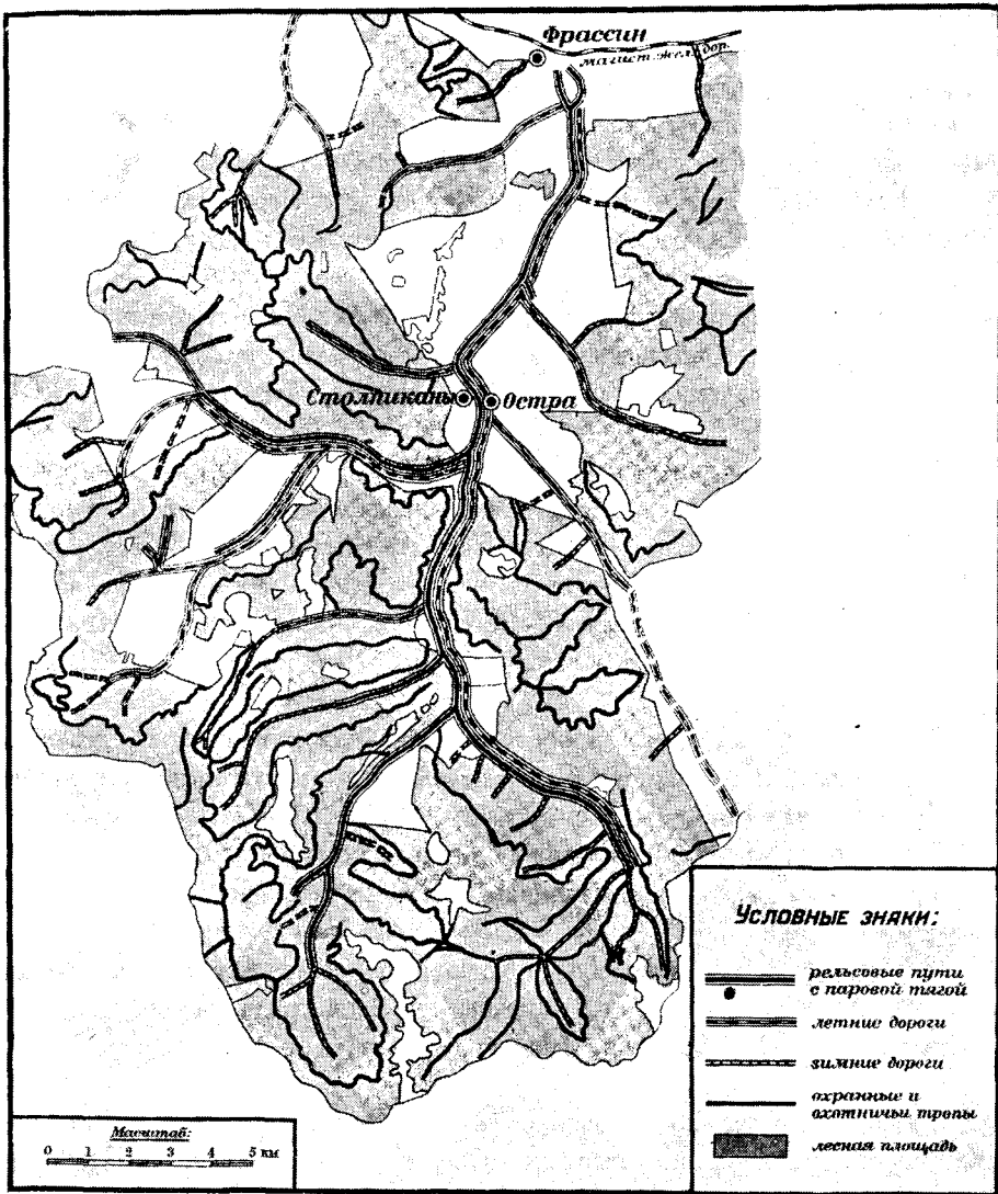
Фиг. 10. План разного рода лесовозных путей в лесной даче.
