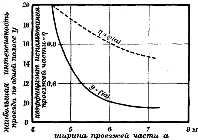
Фиг. 92. Использование проезжей части в зависимости от ее ширины.
