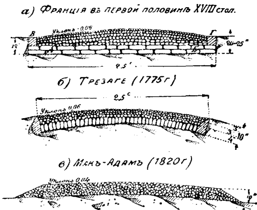
Фиг. 49. Устройство шоссе в XVIII и начале XIX века.
