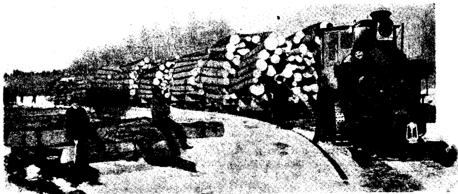
Фиг. 8. Тракторная возка по ледяной колее при малых подъемах.
