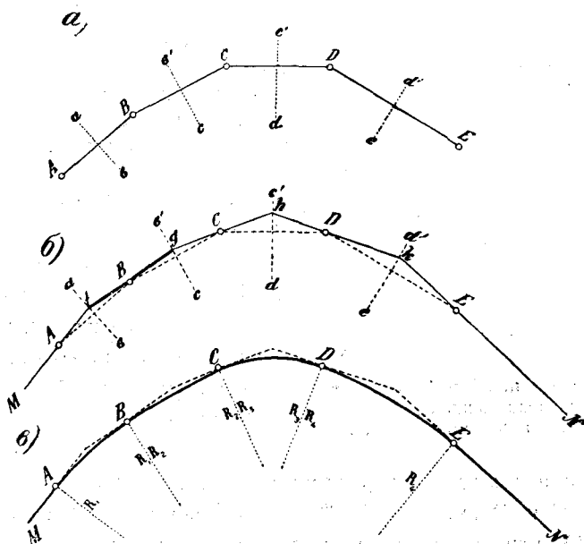
Фиг. 151. Проведение кривой через заданные пять точек A, B, C, D, E .
