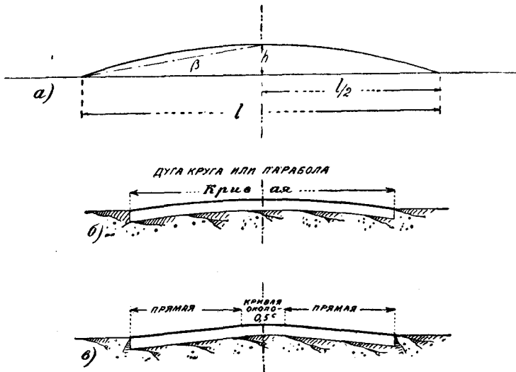
Фиг. 75. Криволинейное и прямолинейное очертание выпуклости проезжей части.
