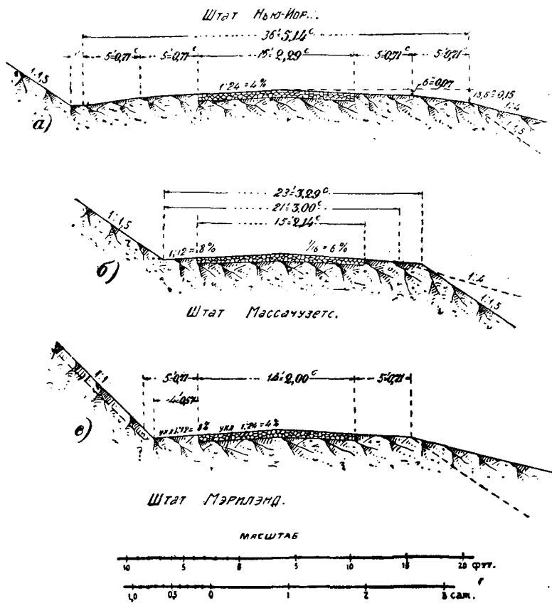
Фиг. 97. Типы прежних американских шоссе для гужевого транспорта.
