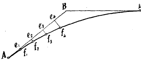
Фиг. 144. Разбивка кривой по ординатам.
