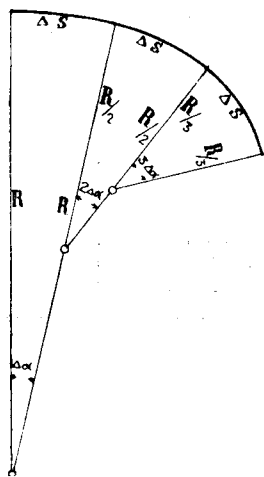
Фиг. 157. Переходная спираль из сопряженных дуг круга.
