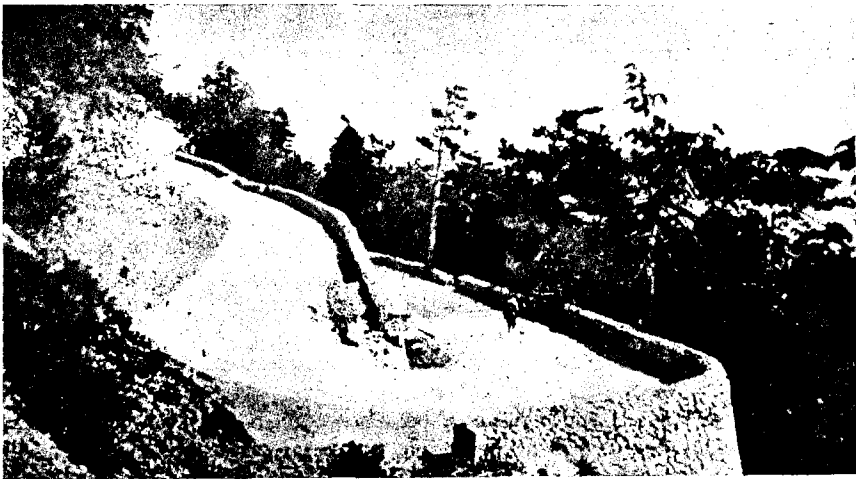
Фиг. 64а. Подъем на Яйлу (Ялта — Бахчисарайское шоссе); серпантина.
