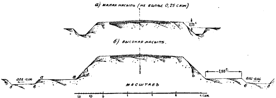
Фиг. 67. Устройство дорожного полотна в насыпи.
