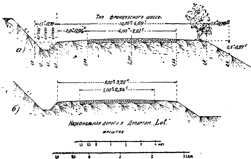
Фиг. 95. Широкие шоссе во Франции.
