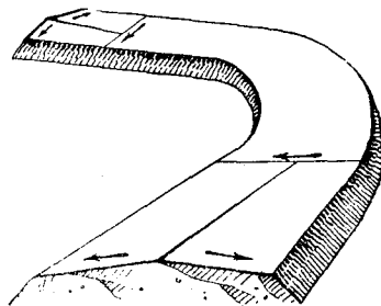
Фиг. 139. Переход от двускатного профиля к односкатному (вираж).
