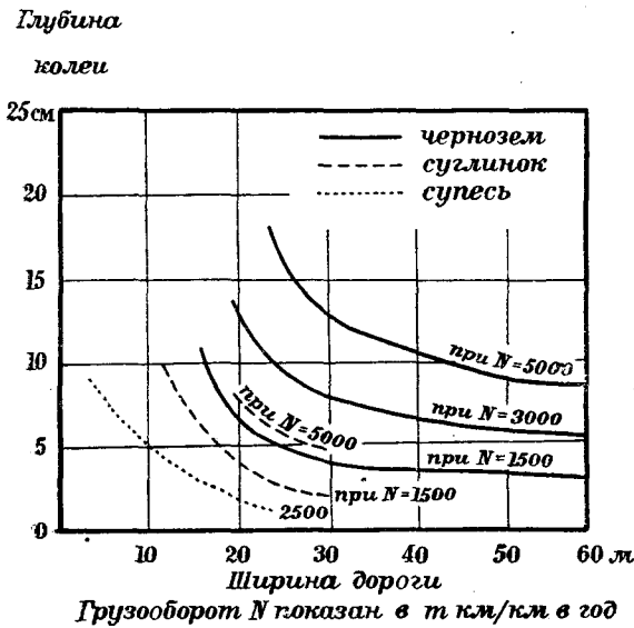
Фиг. 91. Зависимость между шириной грунтовой дороги и глубиной колеи при разных грунтах и грузонапряженности.
