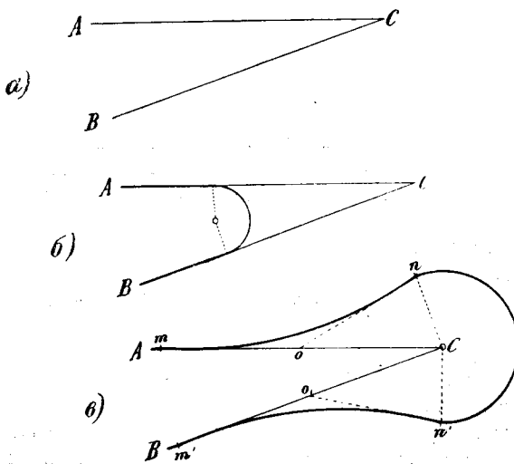
Фиг. 161. Устройство закругления при вершине острого угла.
