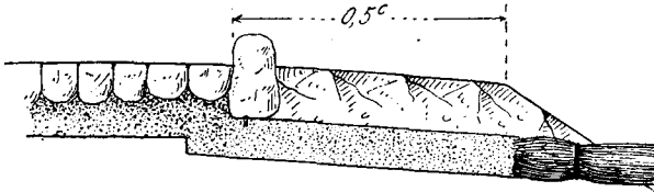
Фиг. 77. Обочина мощеной дороги; оградительный камень и устройство песчаной воронки для осушения основания.
