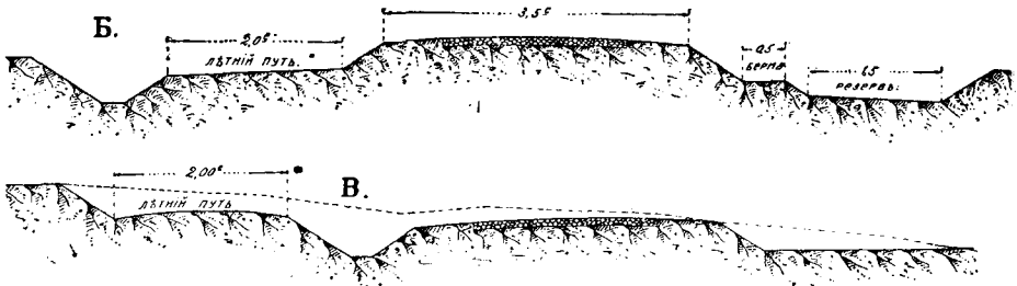
Фиг. 72. Расположение летнего пути и мощеных полос.
