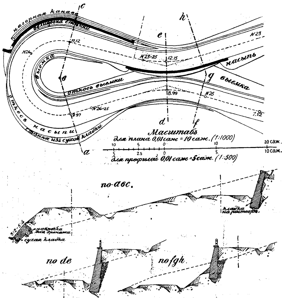
Фиг. 162. План и поперечные профили серпантины.
