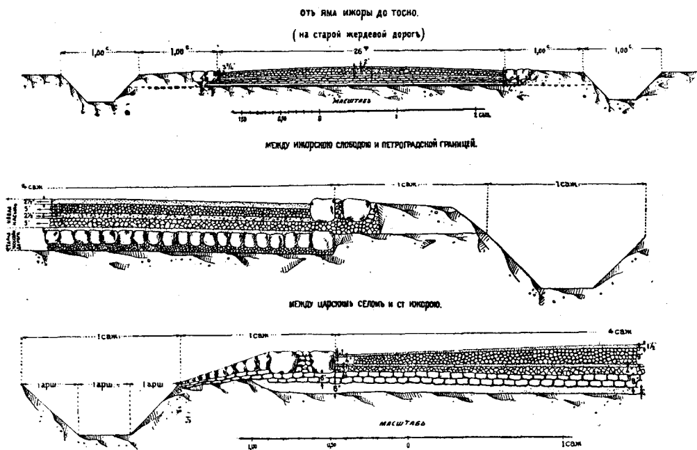
Фиг. 54. Нормальные поперечные профили Московского шоссе 1818 г.
