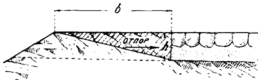
Фиг. 76. Отпорная призма в обочине, удерживающая мостовую.
