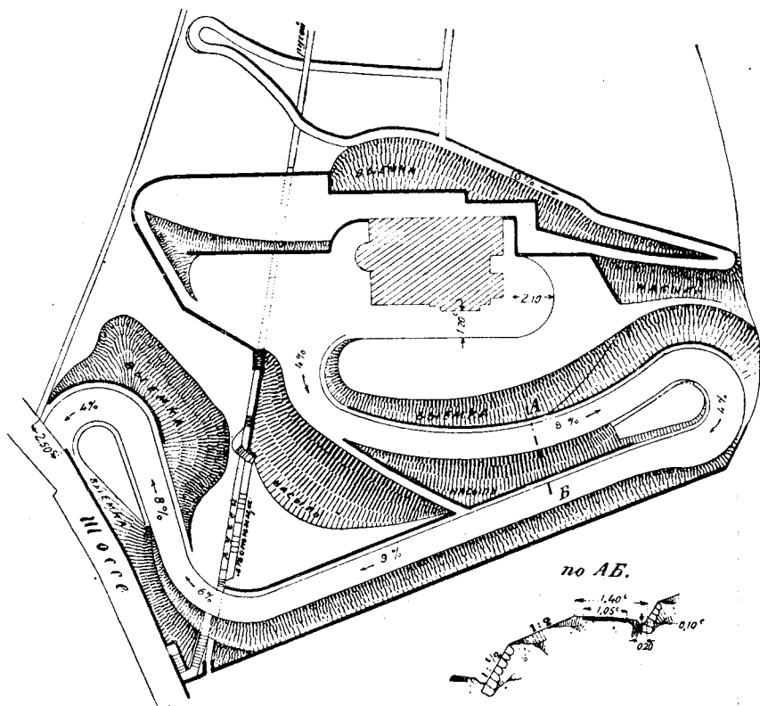
Фиг. 170. Сerpантины для подъезда к зданию на горе (толстые линии обозначают подпорные стены).
