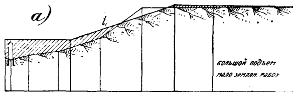
Фиг. 117. Смягчение подъема дороги посредством выемки и насыпи.
