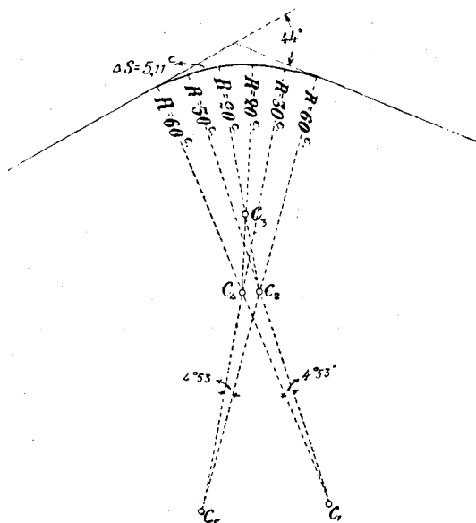
Фиг. 158. Спиральная кривая с переходом от радиуса 150\text{ м} к радиусу 50\text{ м} .
