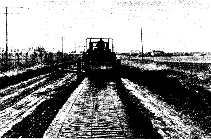
Фиг. 29. Выглаживание грунтовой дороги утюгами и катком.
