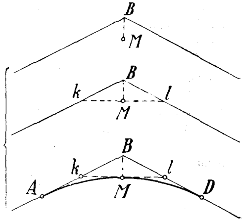
Фиг. 147. Разбивка кривой без таблиц по заданному приближительному положению середины кривой.
